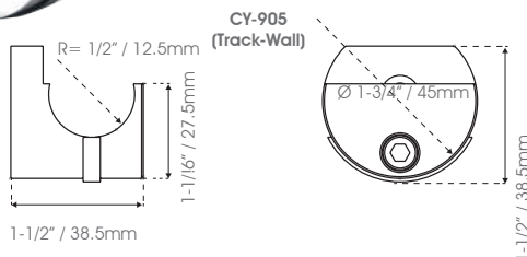
Soporte Tubo-Muro para tubo de 1" (25.4mm) Material: Acero Inoxidable CY-905 Satin ●
