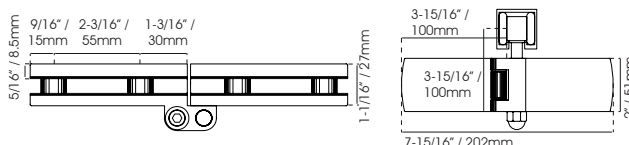
VTR-1410 Bisagra superior con carretilla Cristal-Cristal Satin ●
