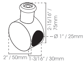
Soporte Tubo-Muro para tubo de 1" (25.4mm) Material: Acero Inoxidable CY-905 Satin ●
