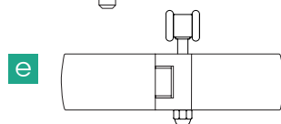
VTR-1410 Bisagra superior con carretilla cristal-cristal
