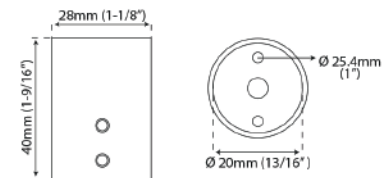
Soporte interior tubo-cristal para tubo de 1" (25.4mm) Material: Acero Inoxidable CY-910 Satin ● CY-945 Satin ●
