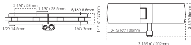
VTR-1412 Bisagra inferior con guía Cristal-Cristal Satin ●
