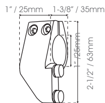
Tope para tubo de 1" (25.4mm) Material: Acero Inoxidable CY-924SS Satin ●
