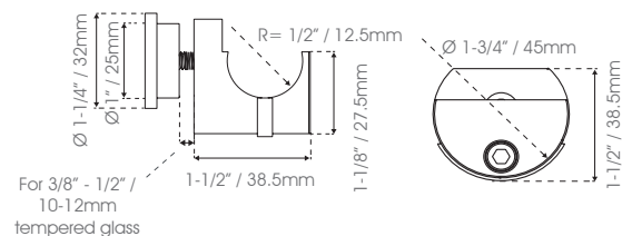
Soporte Tubo-Cristal para tubo de 1" (25.4mm) Material: Acero Inoxidable CY-906 Satin ●
