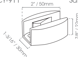
Guía Ajustable para puerta de cristal / Espesor de cristal 5/16" - 1/2" (8-12mm) Material: Acero Inoxidable CY-911 Satin ●
