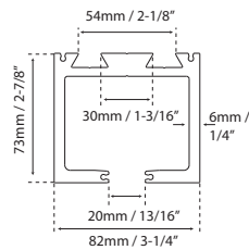
JK15550 Riel superior e inferior con pinzas / Aluminio
